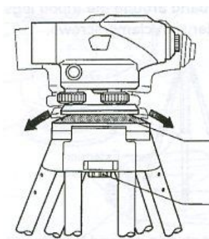
Площадка штатива
